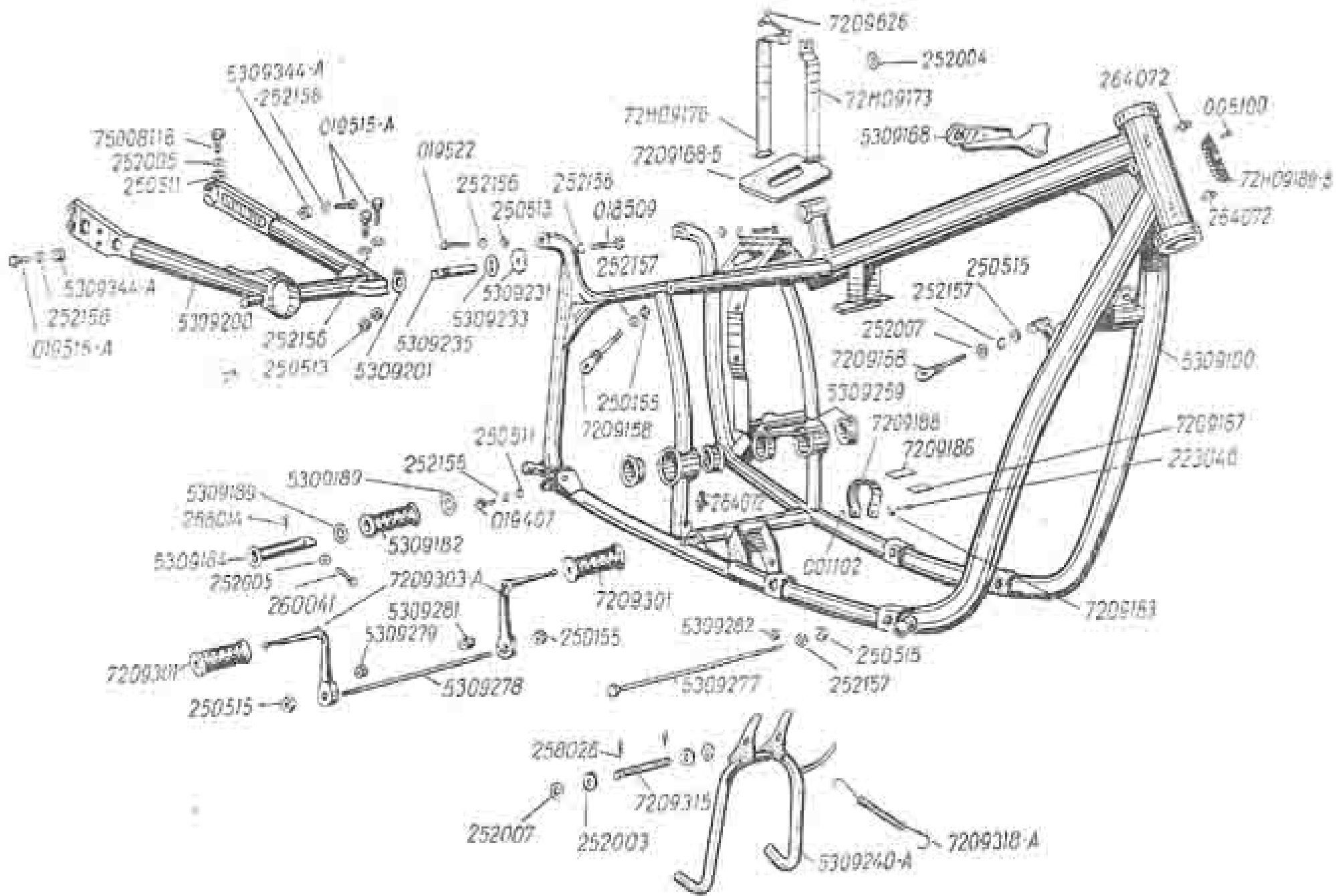
Рис. 19. Разд. подставка, подножии
