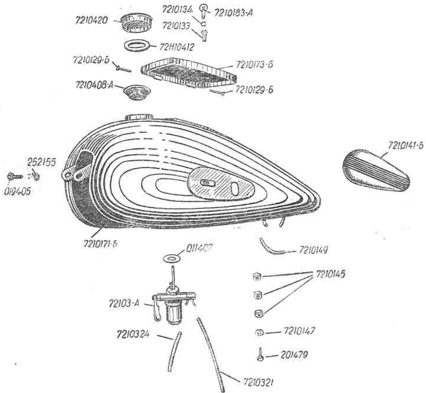
Рис. 24. Бензобак
