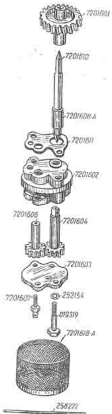
Рис. 7. Масляный насос
