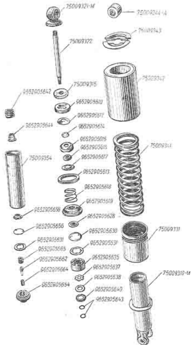
Рис. 21. Амортизатор рамы
