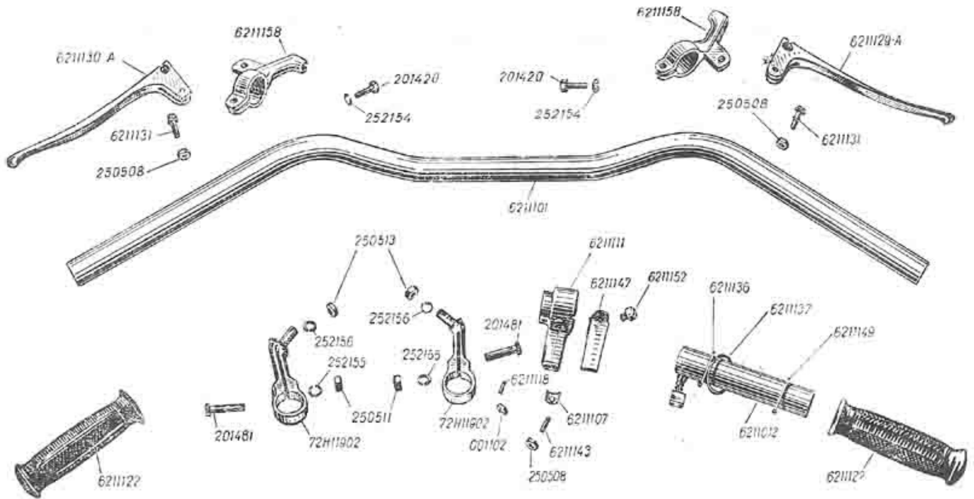
Рис. 25. Руль, рычаги, рукоятки управления
