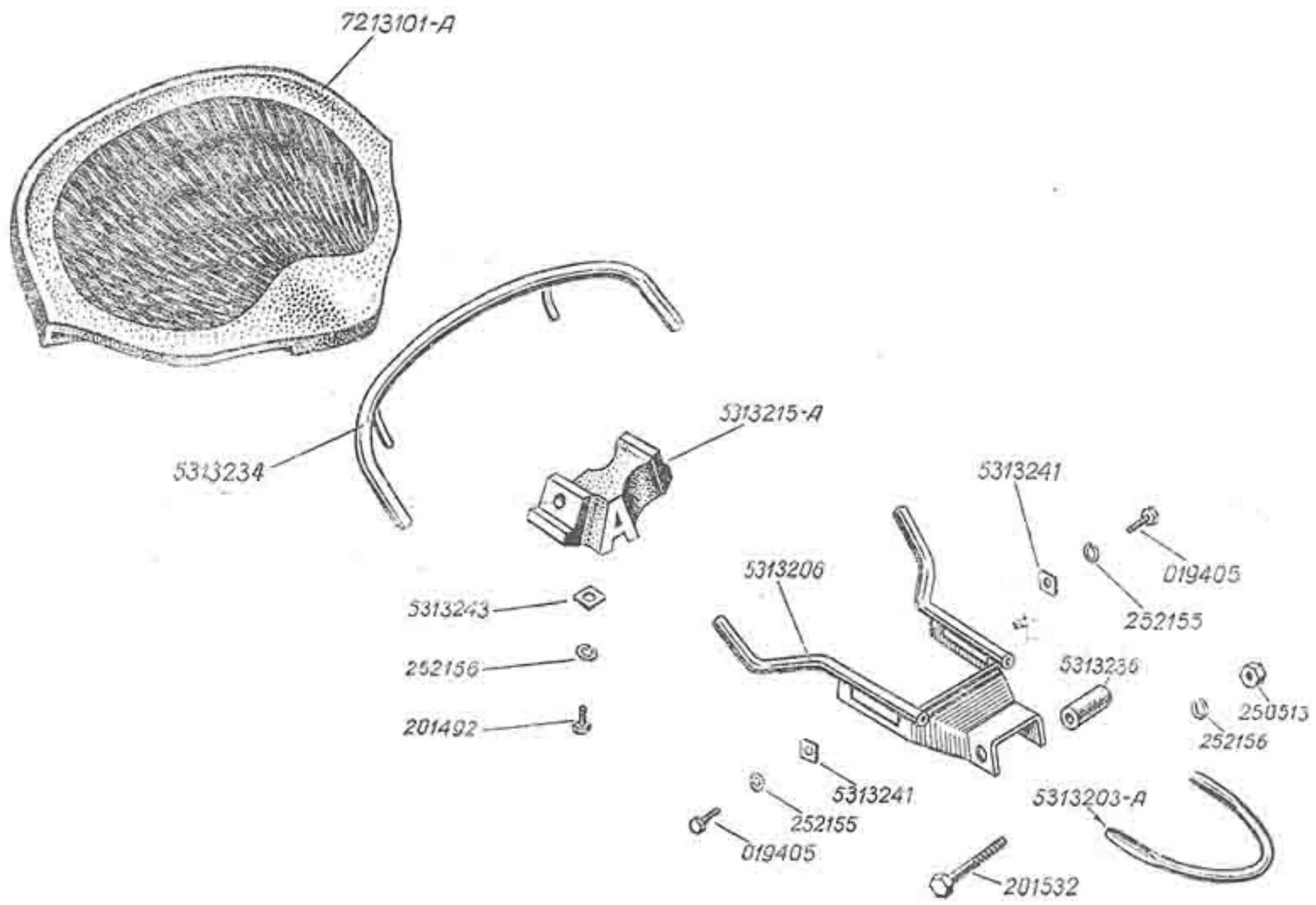
Рис. 29. Седло переднее
