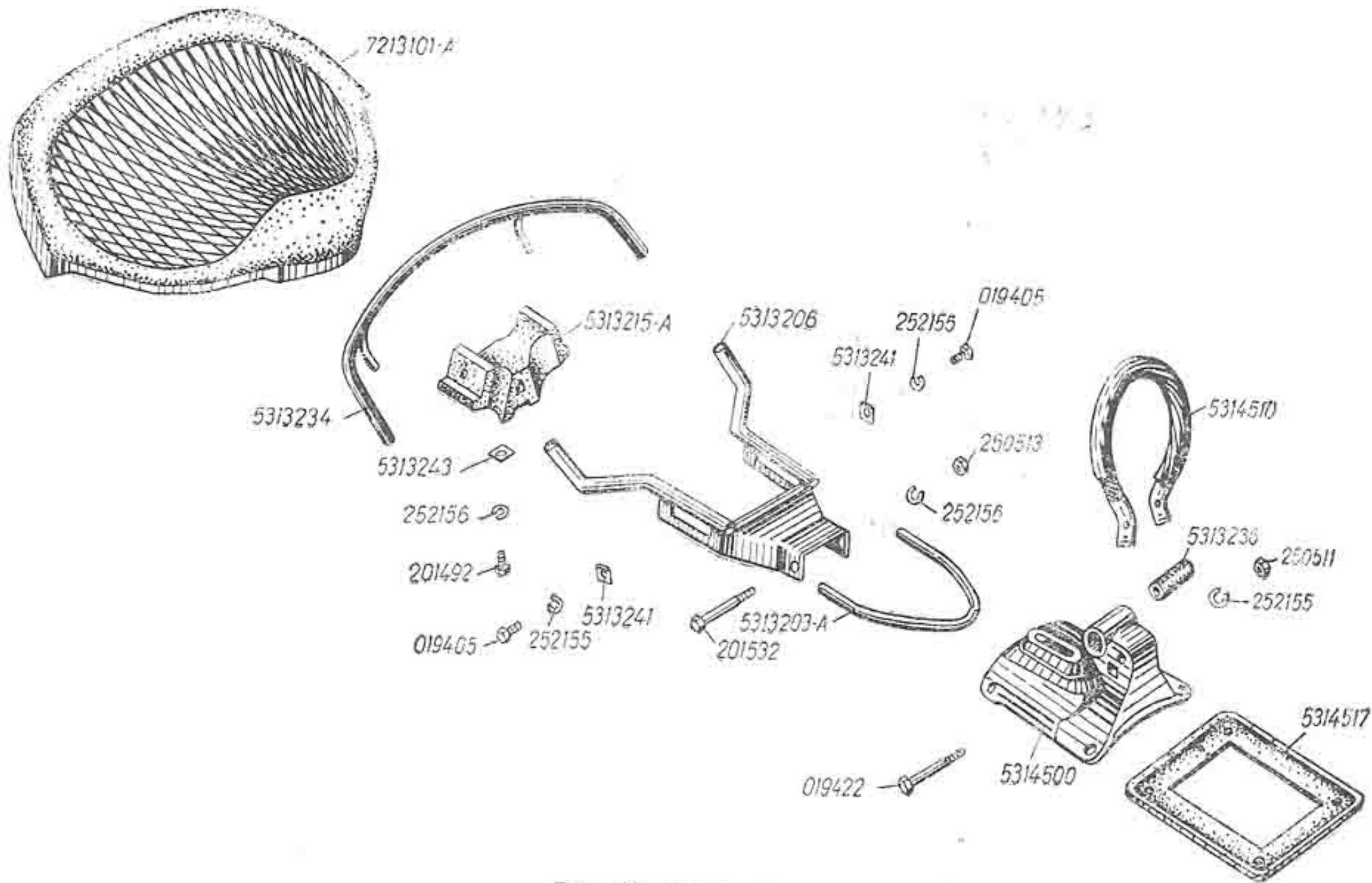
Рис. 30. Седло заднее
