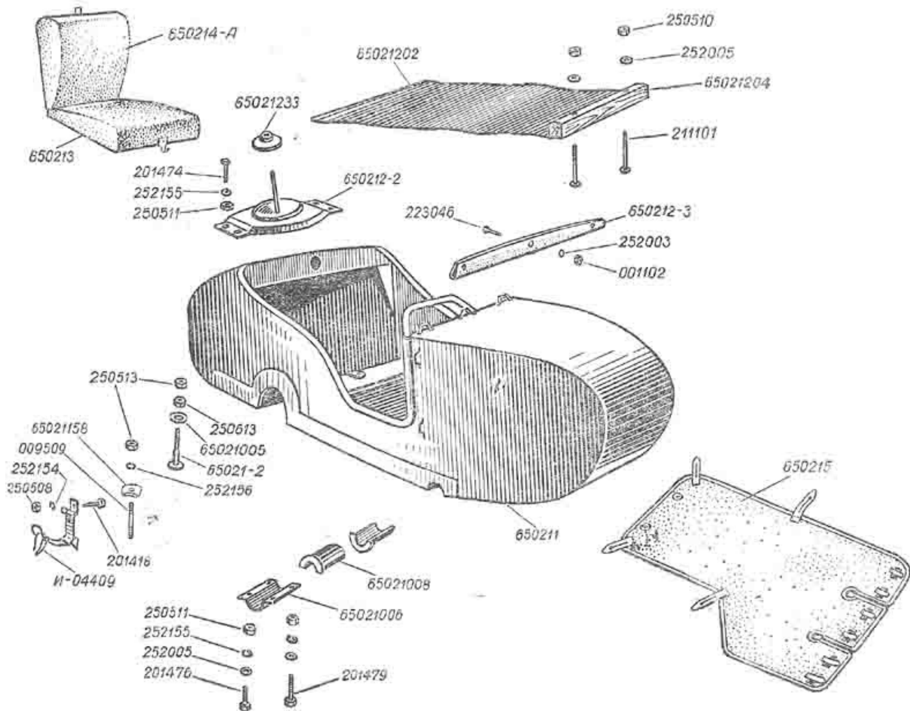
Рис. 37. Кузов коляски
