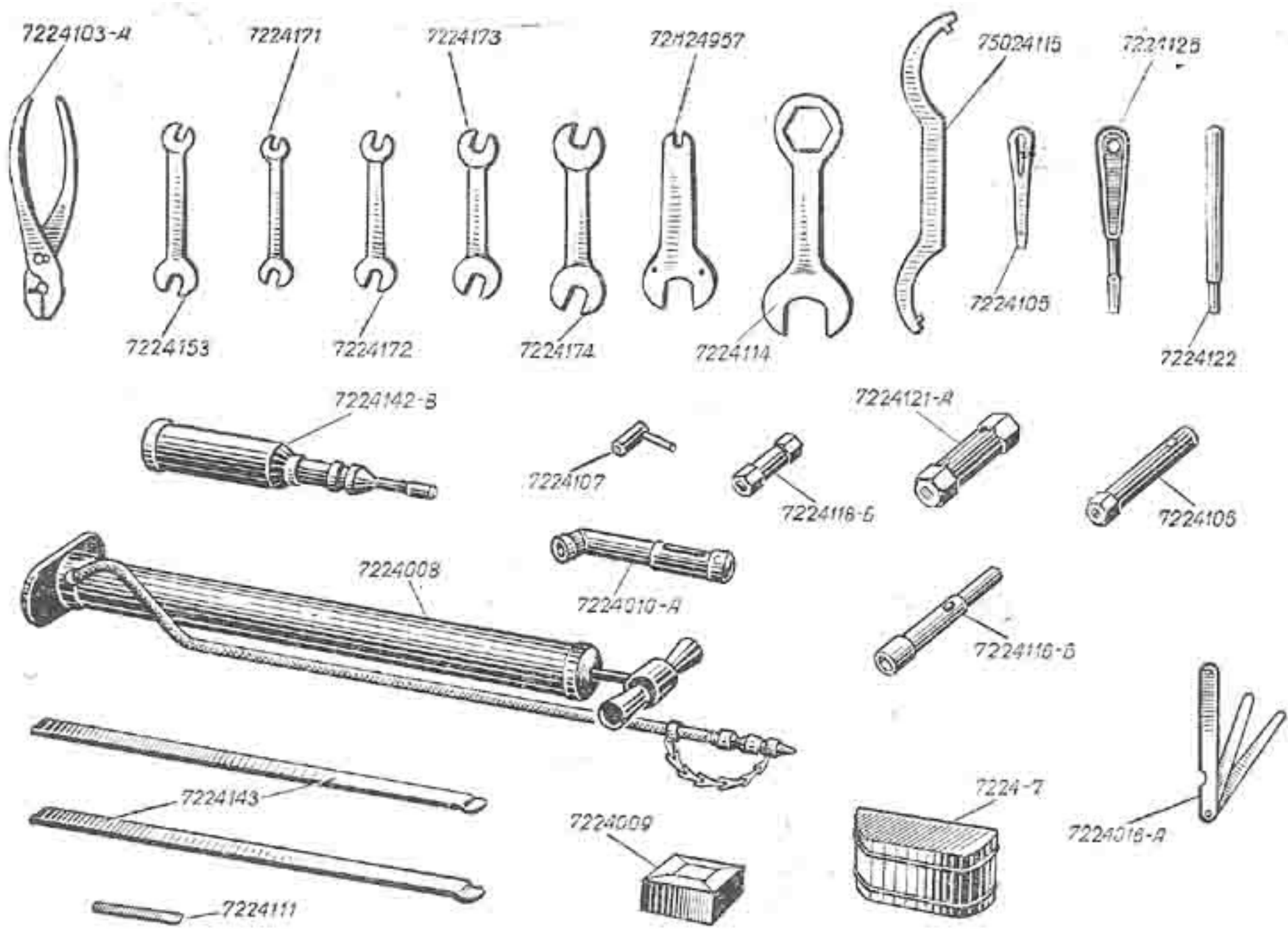
Рис. 38. Инструменты водителя
