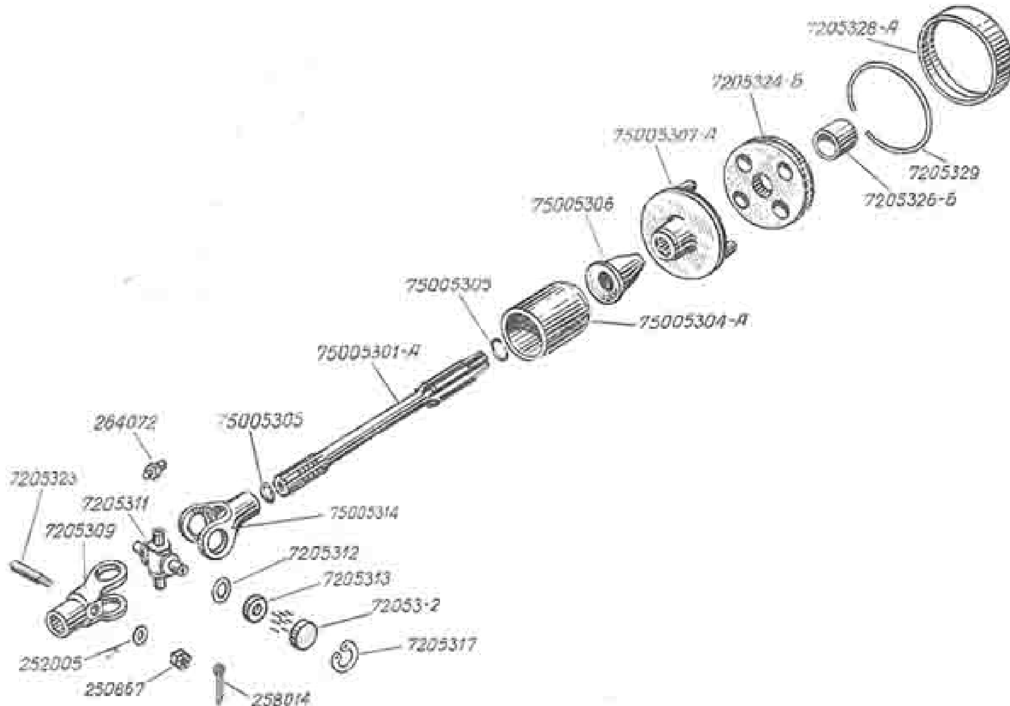
Рис. 15. Карданный вал
