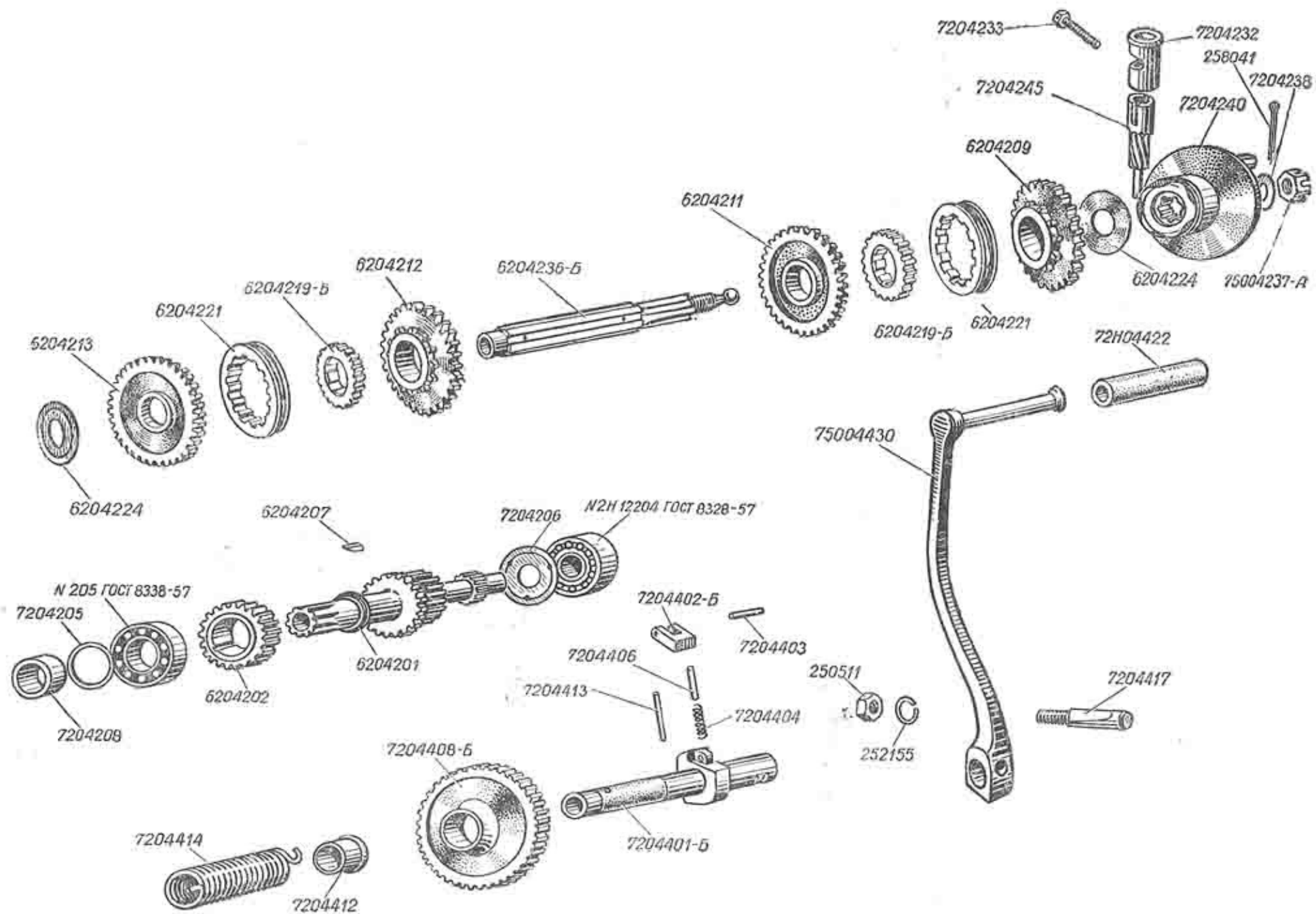
Рис. 11. Валы и шестерни коробки передач
