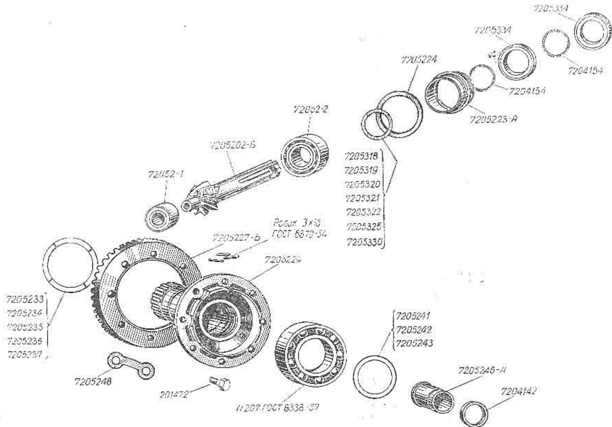
Рис. 14. Редуктор главной передачи
