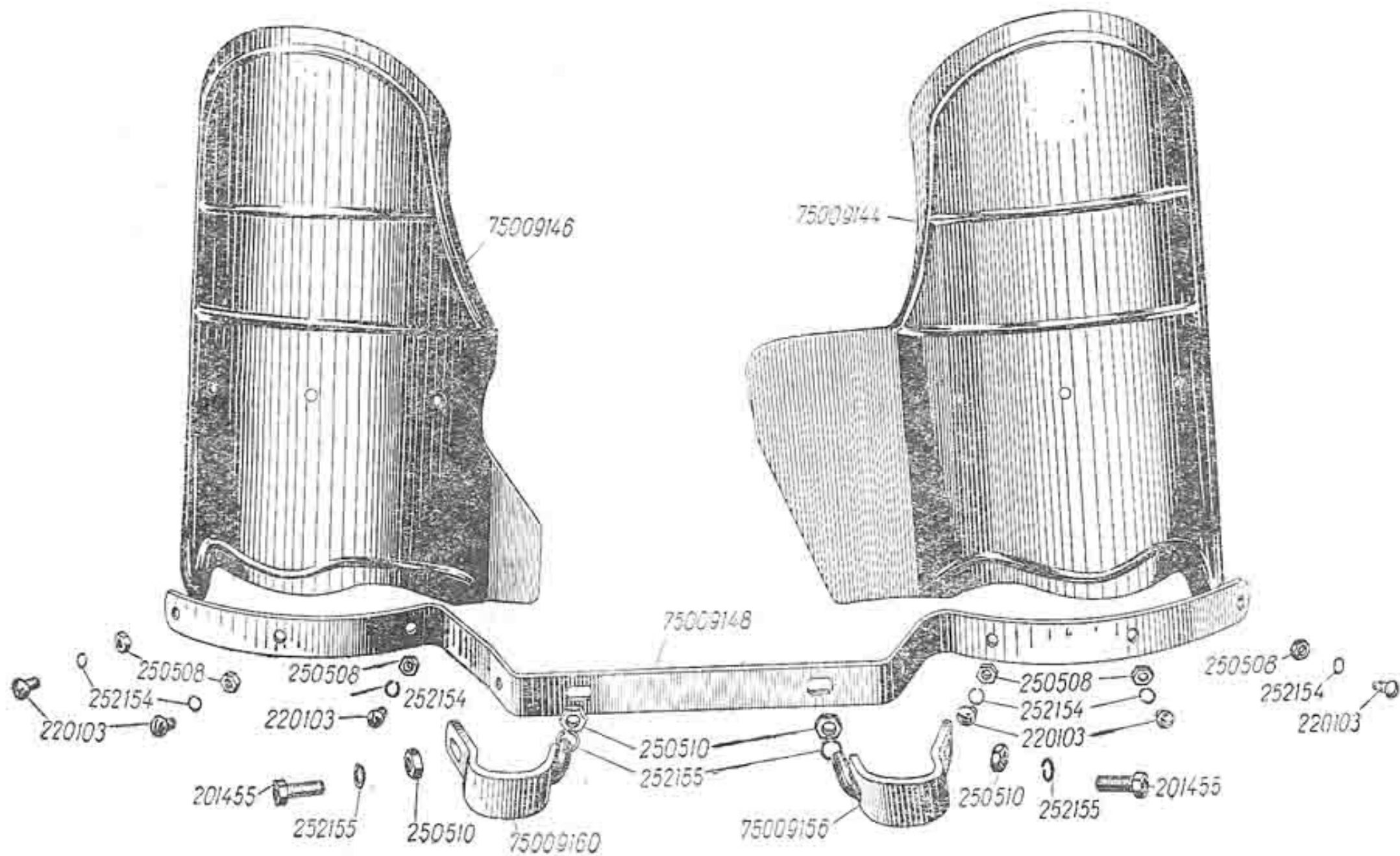
Рис. 23. Брызговики
