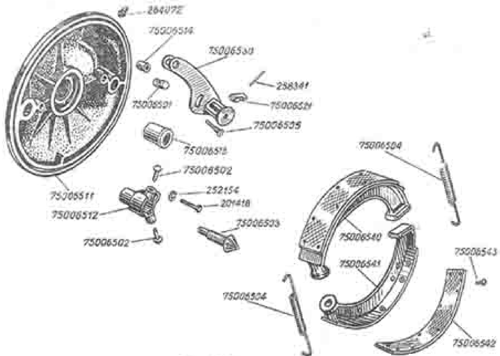
Рис. 17. Тормоз передний
