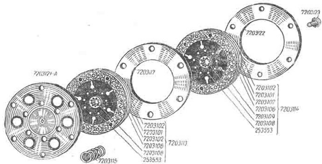
Рис. 8. Сцеplение
