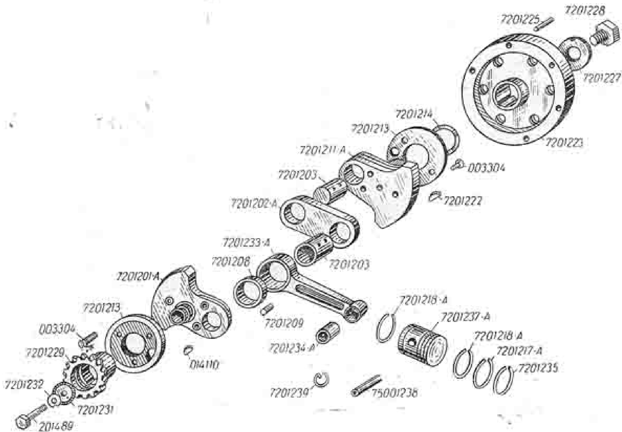
Рис. 4. Коленчатый вал с шатунами и поршнями
