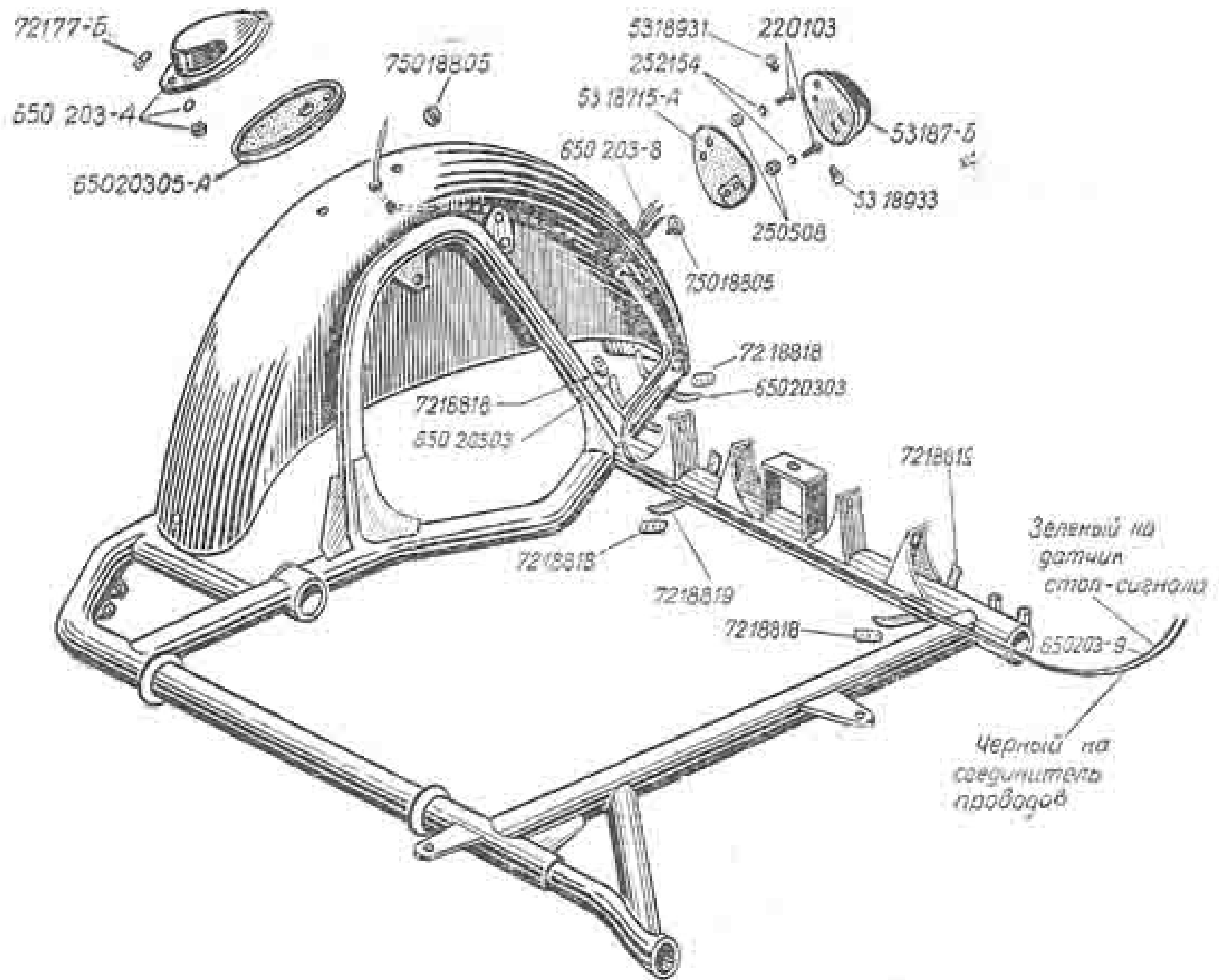
Рис. 36. Монтажная схема электрооборудования коляски.
