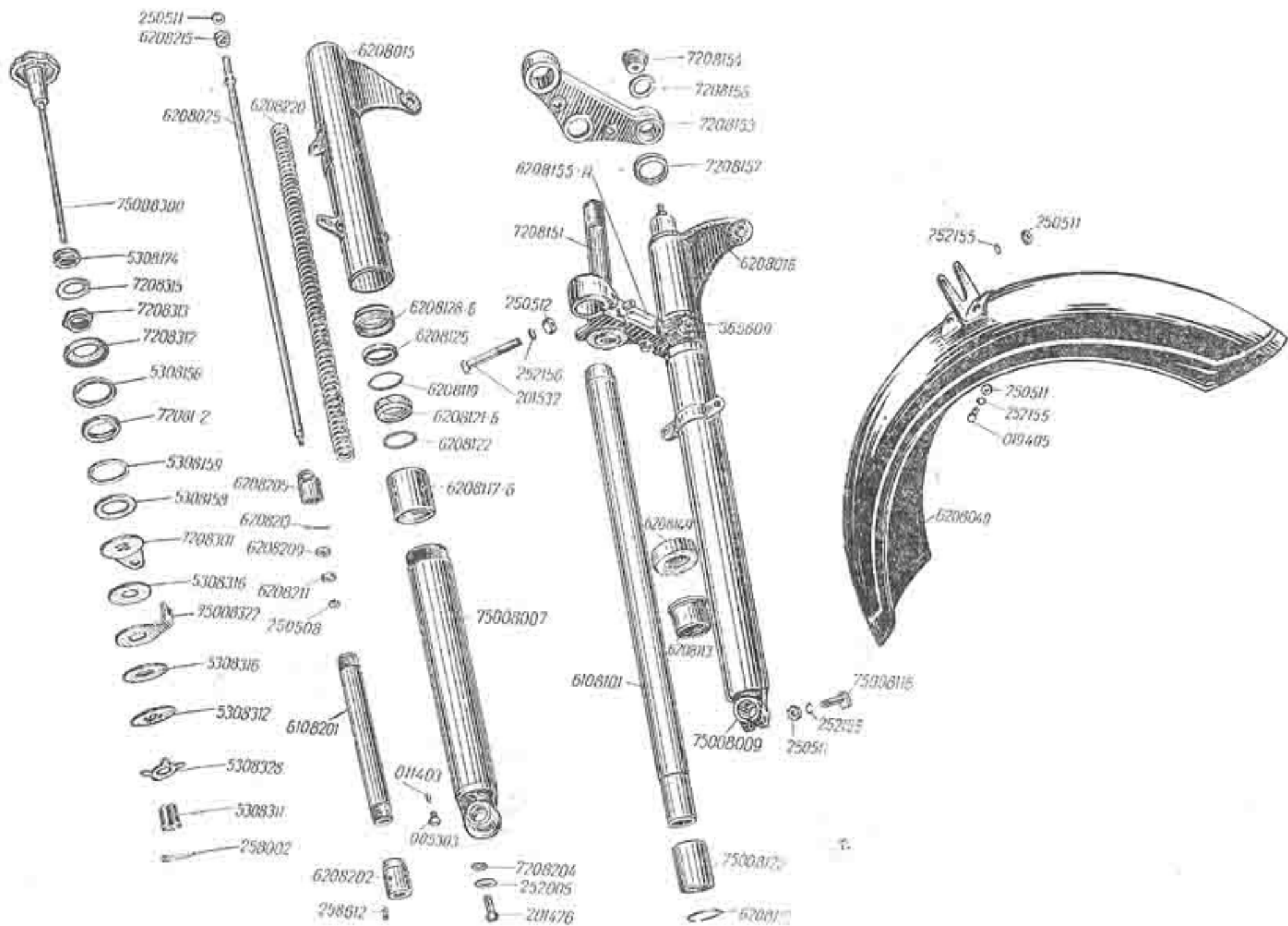
Рис. 18. Вилка передняя
