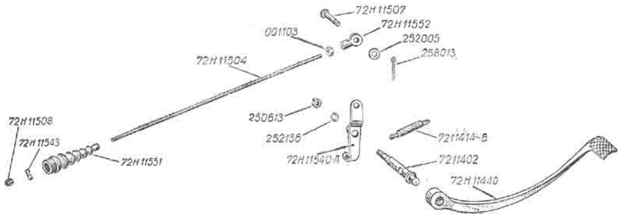
Рис. 27. Привод заднего тормоза
