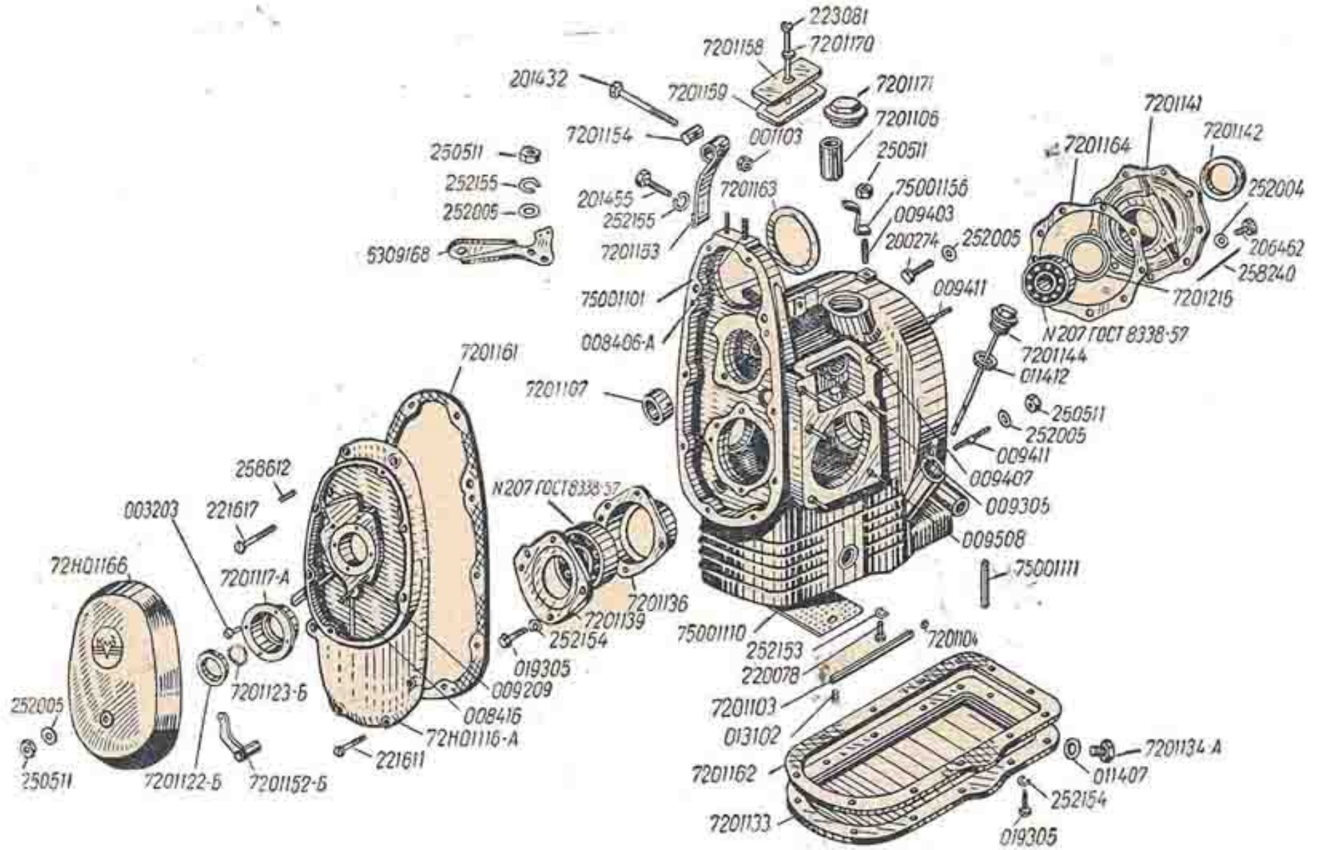
Рис. 3. Картер двигателя с крышками и поддоном
