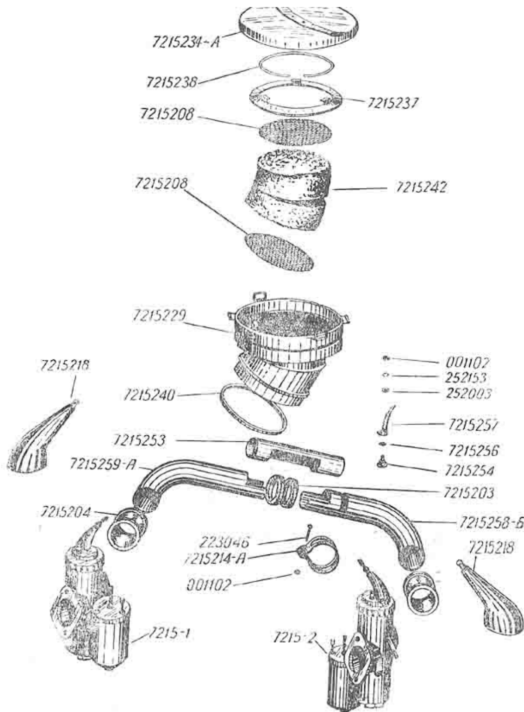
Рис. 31. Карбюраторы, корректор, воздушный фильтр
