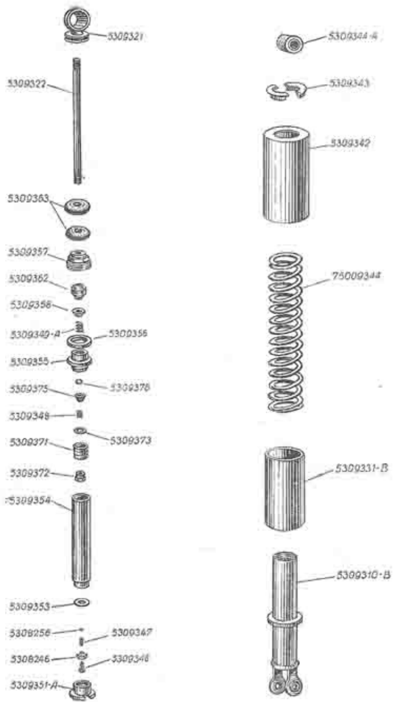
Рис. 20. Агрегатное устройство
