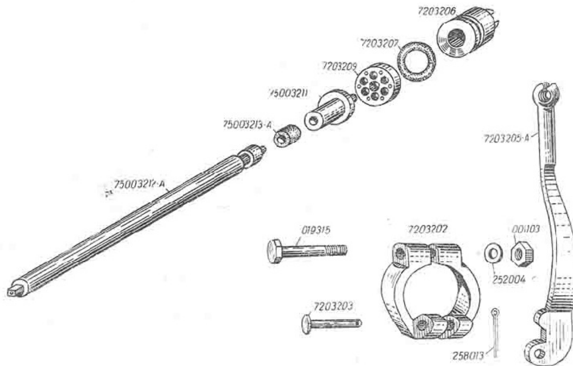
Рис. 9. Механизм выключения сцеplения
