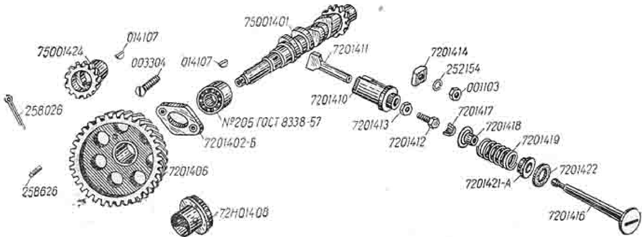
Рис. 6. Механизм газораспределения
